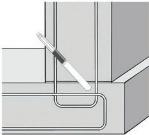
Bohrung im 45° Winkel
